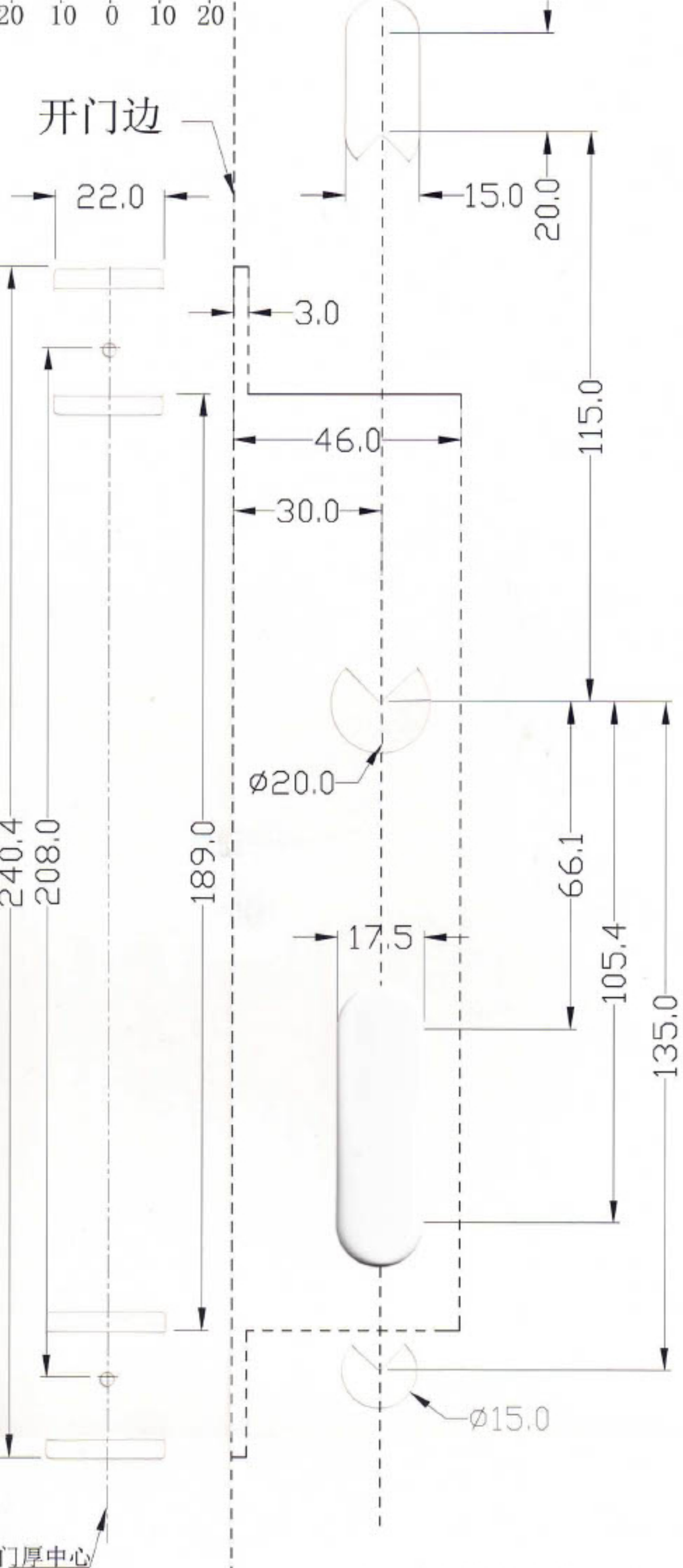
RX-ODS开孔模板 (30*85)
