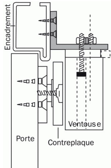
Cas n° 2 : porte tirante, équerre en L :
